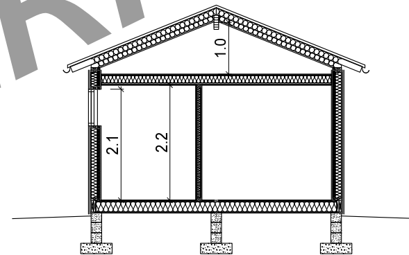
Sektion B-B
